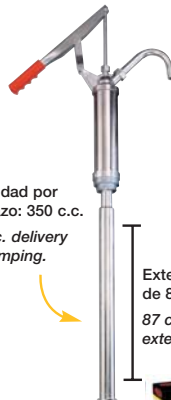
Bomba Extractora para Tambo Barrel Pump
